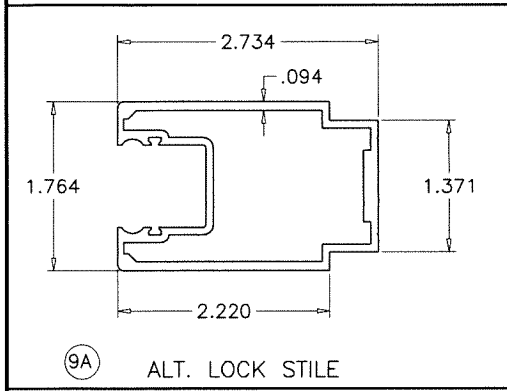
9 LOCK STILE
